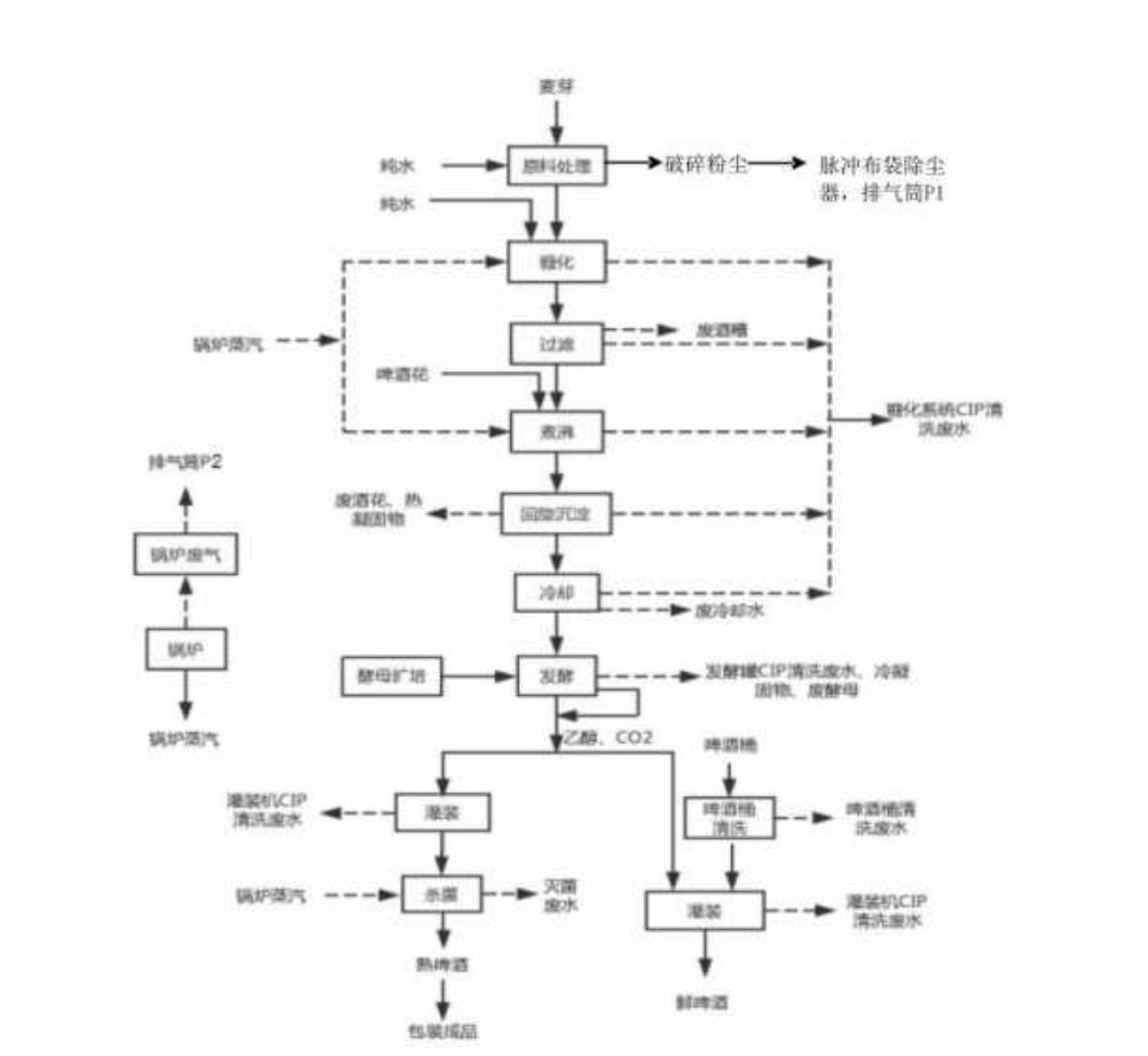
图 3-14 啤酒生产工艺流程图
