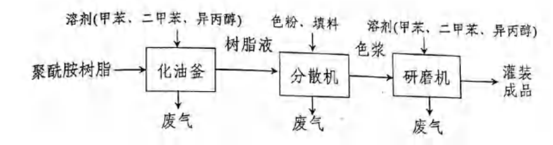
图 3-16 溶剂型塑料油墨工艺流程图
