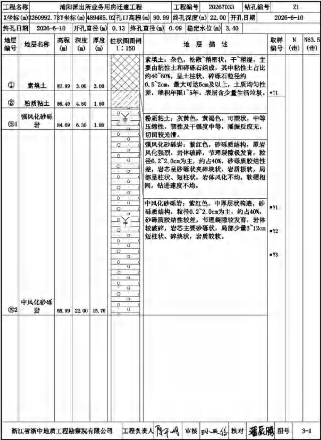
图 3-8 钻孔柱状图
