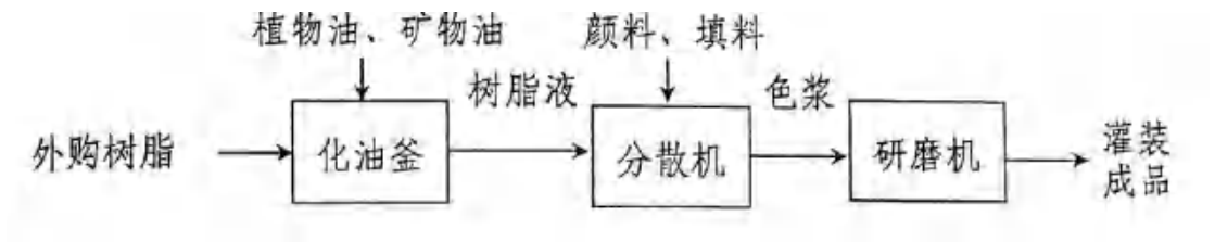
图 3-17 平版油墨工艺流程图
