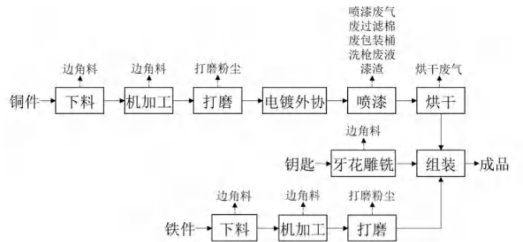
图 3-18 生产线工艺流程图
