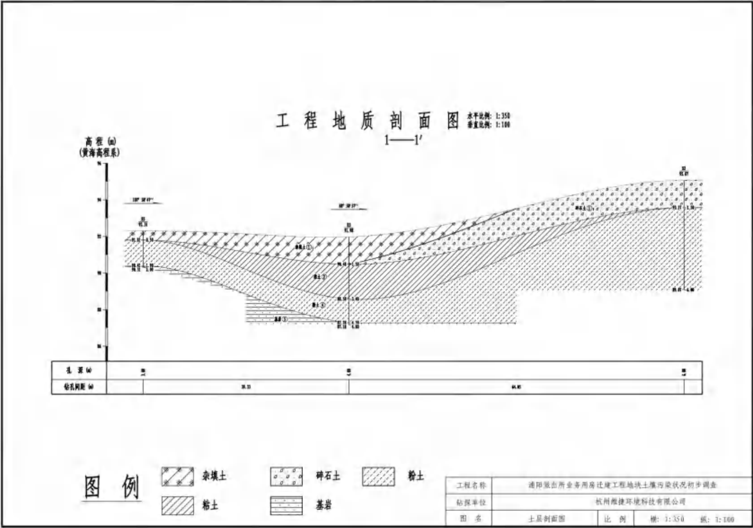
图 6-2 土层剖面图 (1-1' )
