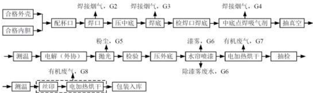
图 3.3-19 外壳和内胆装配工艺流程图
