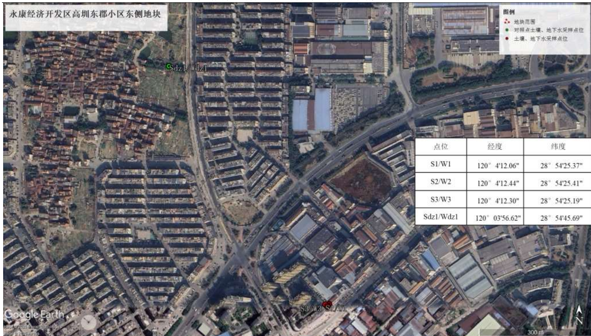
图 4.1-2 采样布点图（含对照点）
