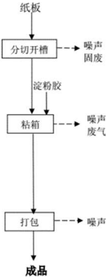
图 3.3-9 印刷产品生产工艺流程图
