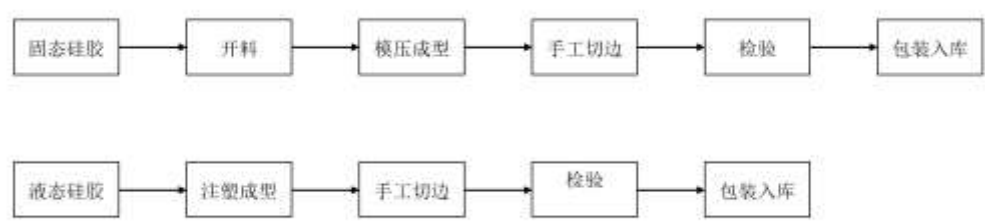
图 3.3-21 生产工艺流程图
