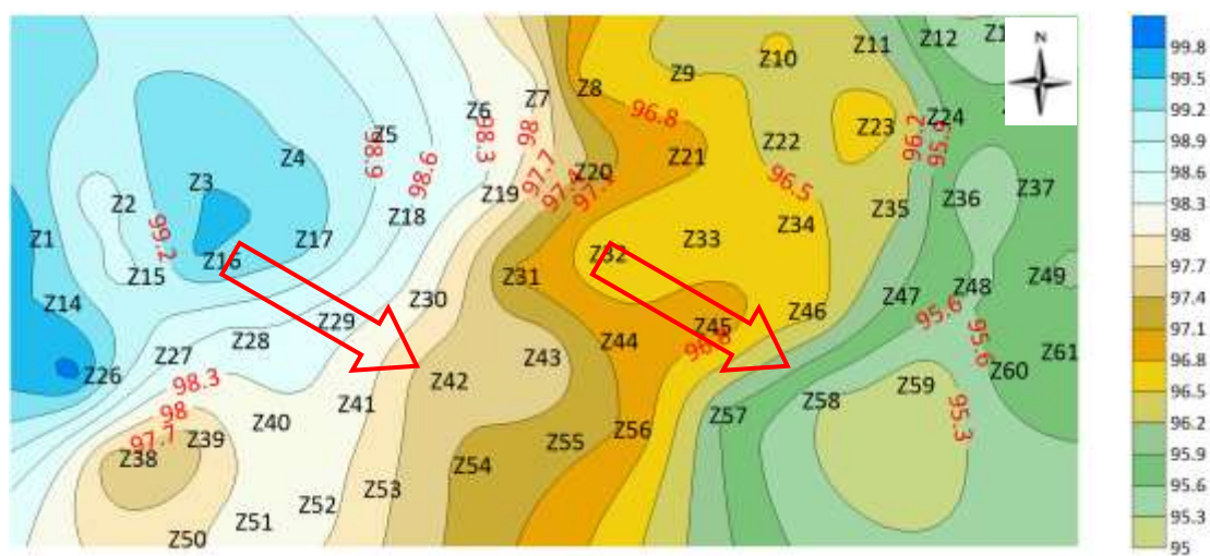
图 3.2-8 引用地块地下水等水位线图
