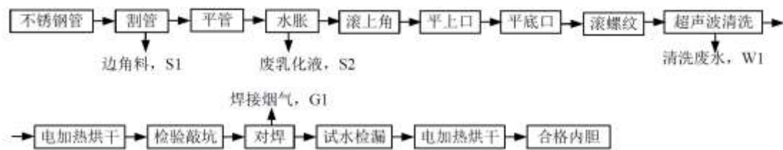
图 3.3-18 内胆生产工艺流程图
