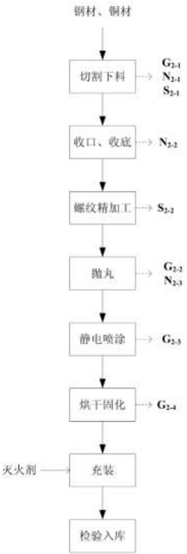
图 3.3-23 生产工艺流程图
