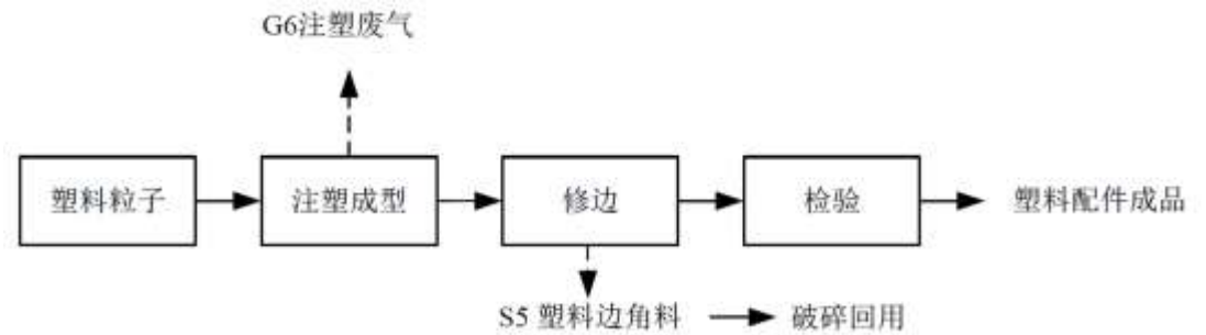
图 3.3-20 塑料配件生产工艺流程图
