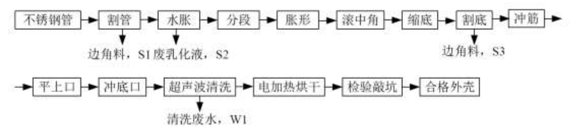
图 3.3-17 外壳生产工艺流程图
