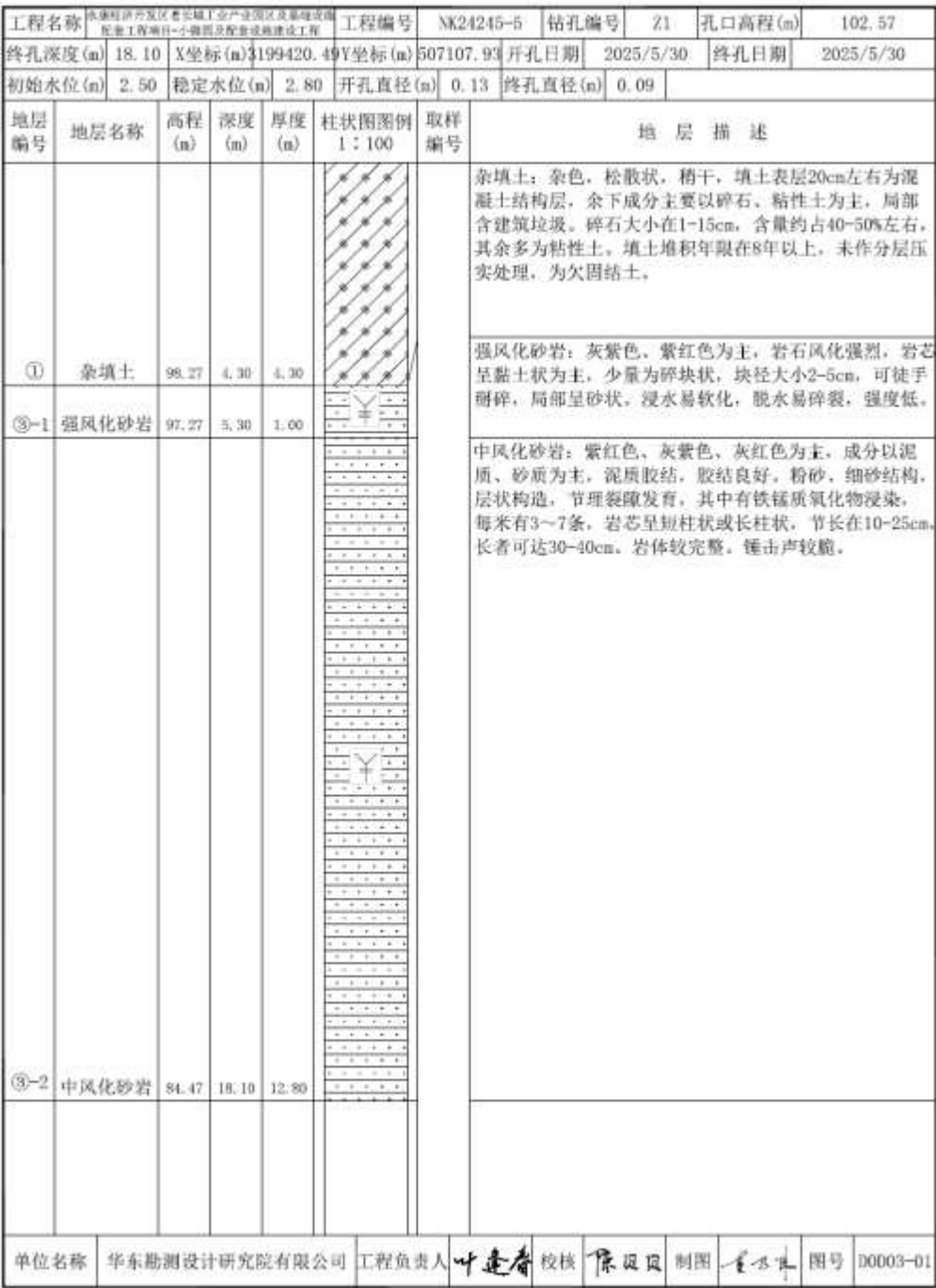
图 3.2-7 钻孔柱状图
