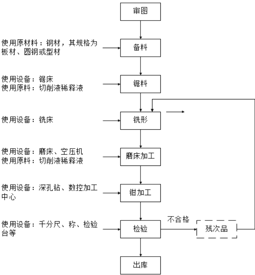
图 3.3-7 生产工艺流程图
