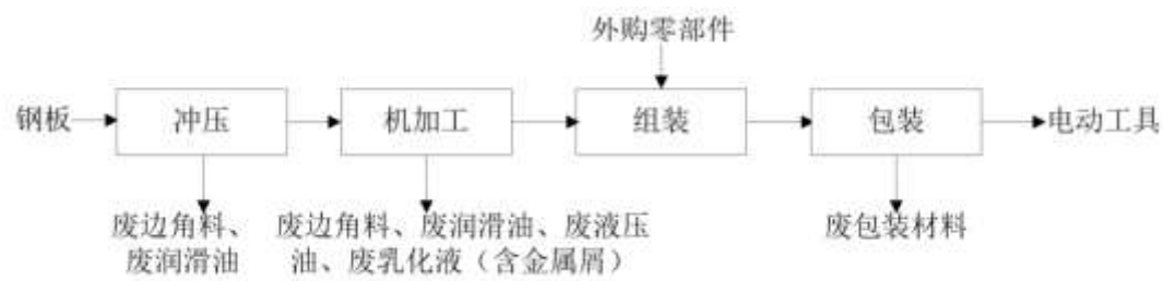
图 3.3-14 生产工艺流程图
