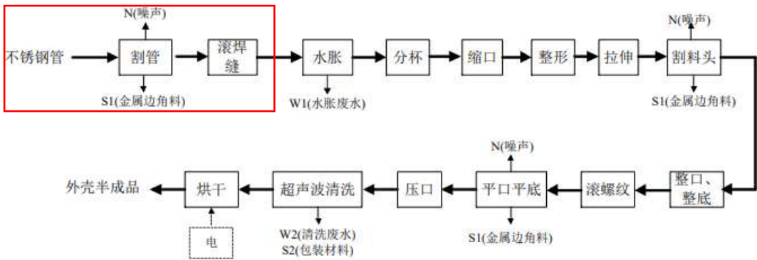
图 3-23 生产工艺流程图
