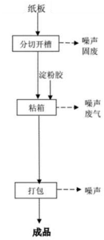
图 3-38 生产工艺流程图
