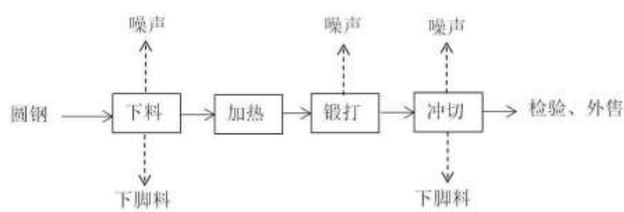
图 3-27 生产工艺流程图
