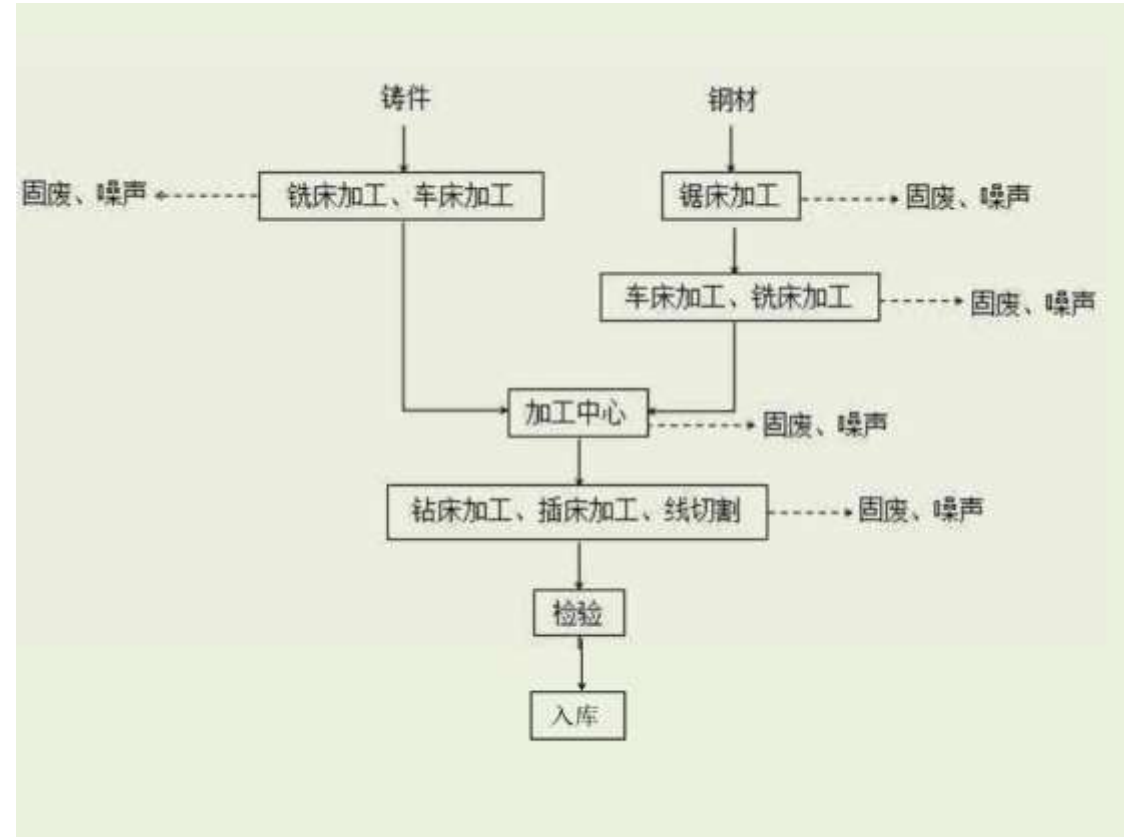
图 3-20 生产工艺流程图
