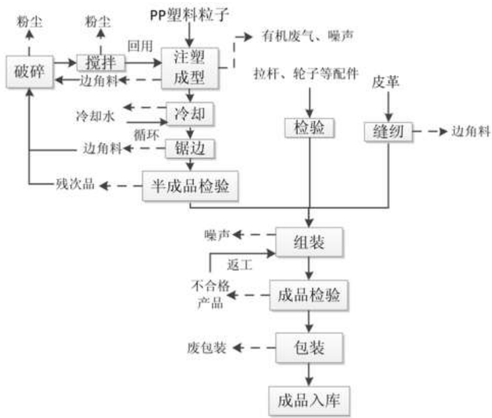
图 3-18 生产工艺流程图
