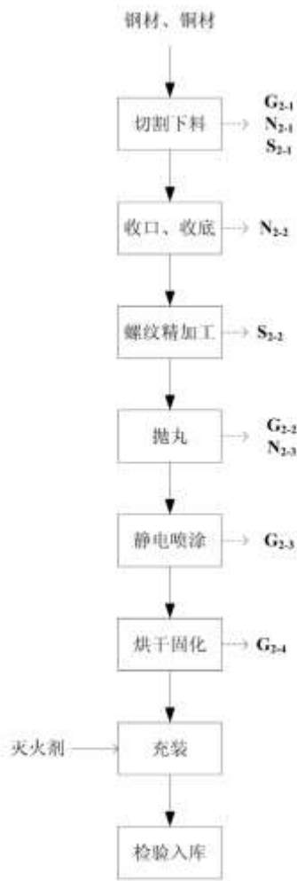
图 3-29 生产工艺流程图
