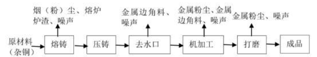
图 3-22 生产工艺流程图
