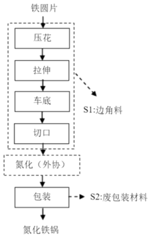
图 3-21 生产工艺流程图
