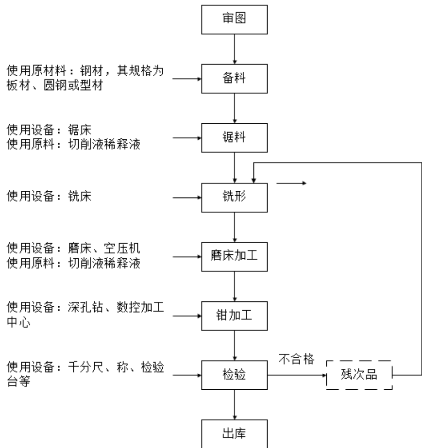
图 3-17 生产工艺流程图
