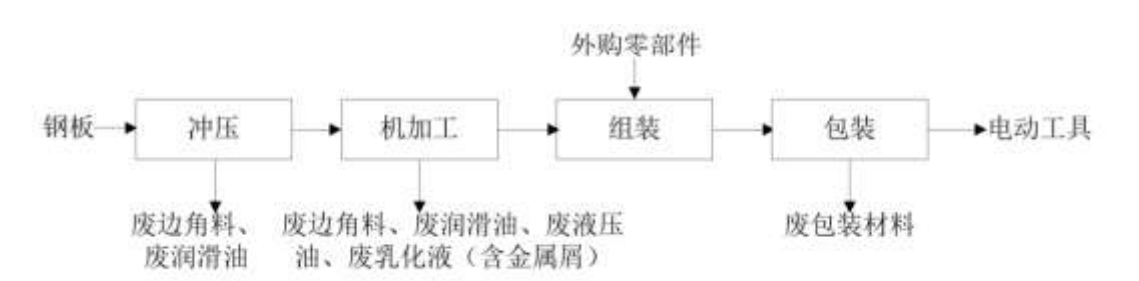
图 3-14 生产工艺流程图
