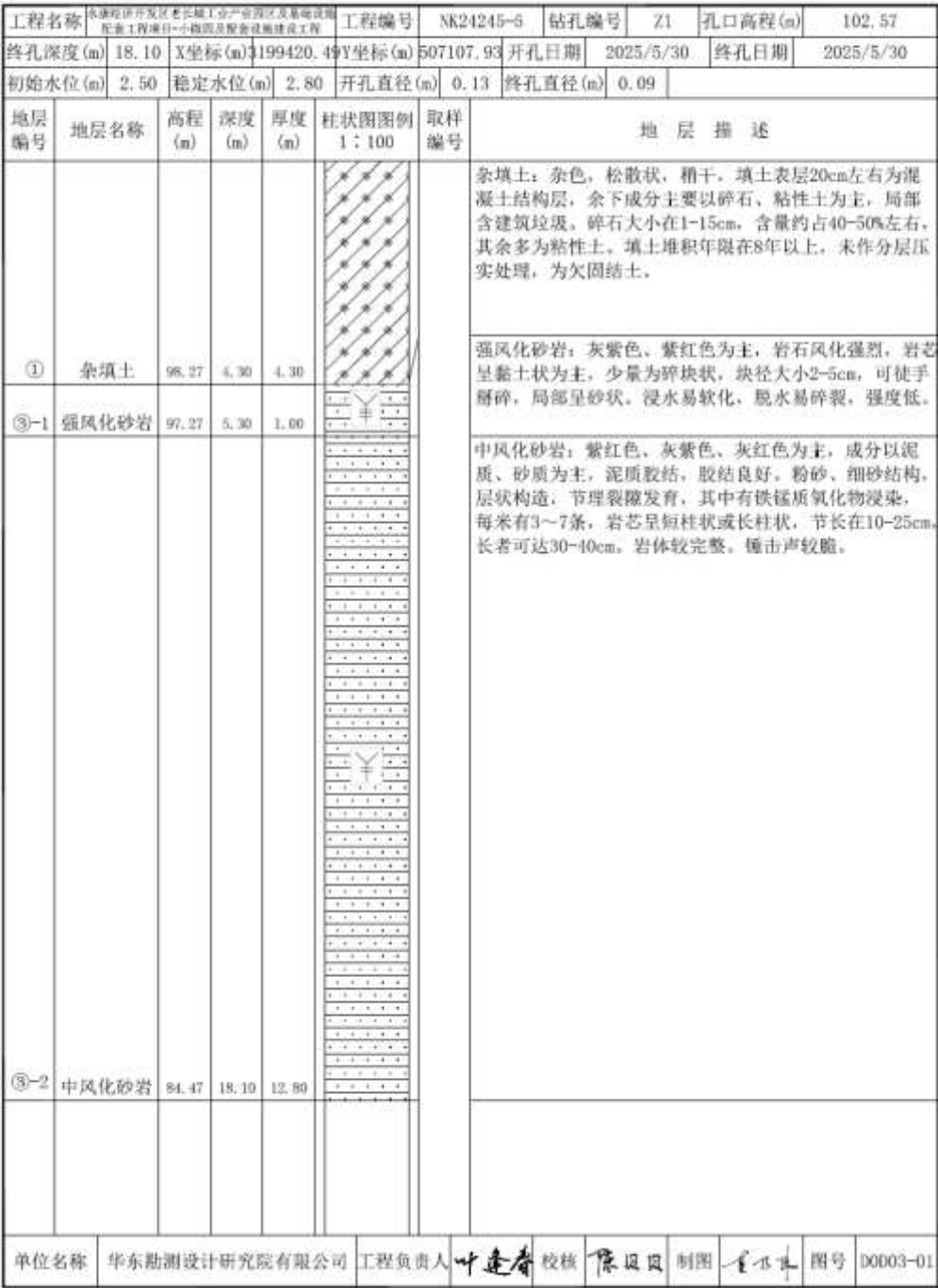
图 3-9 钻孔柱状图
