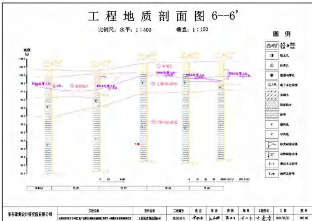
图 3-10 地质剖面图
