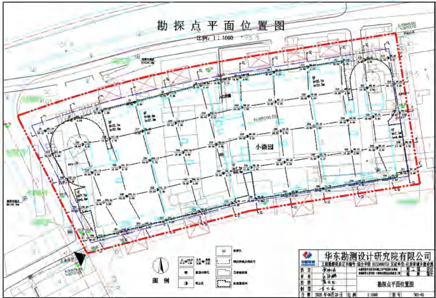
图 3-8 地勘地块勘探平面图
