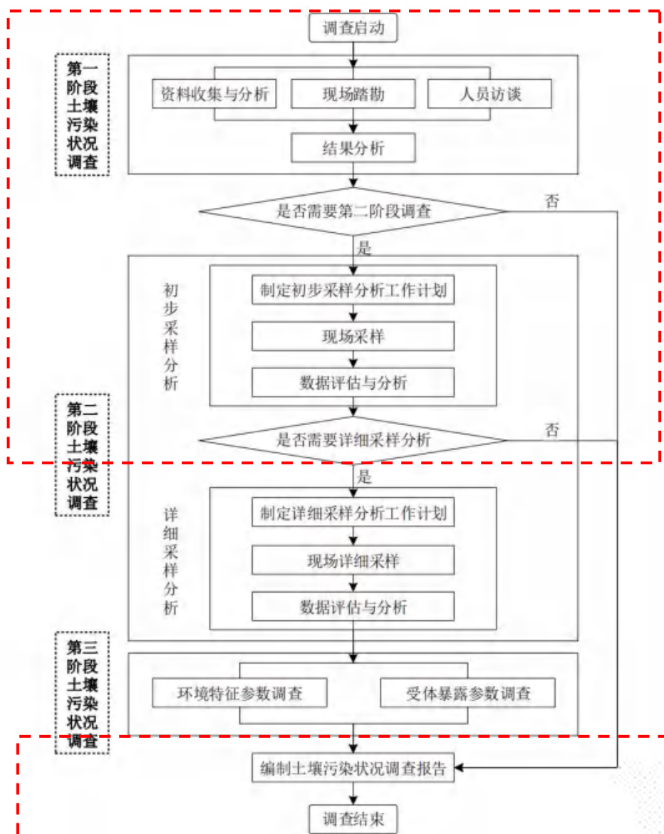
图 2-2 永康市造漆厂地块土壤污染状况调查流程图（红框内为本次调查流程）
