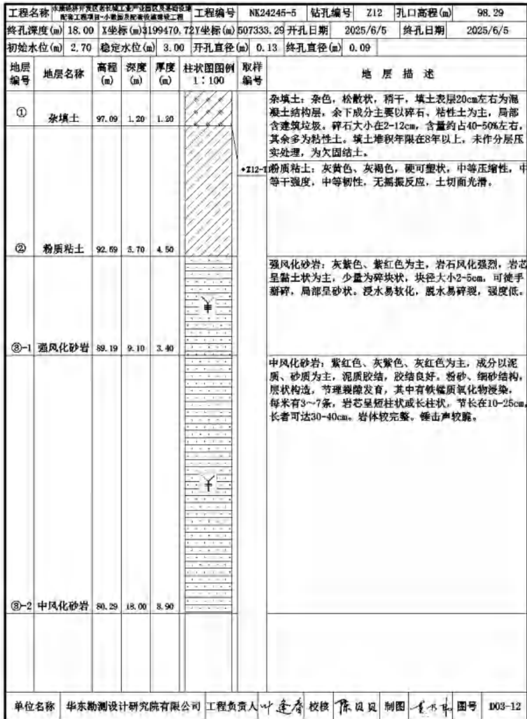
图 3-9 钻孔柱状图
