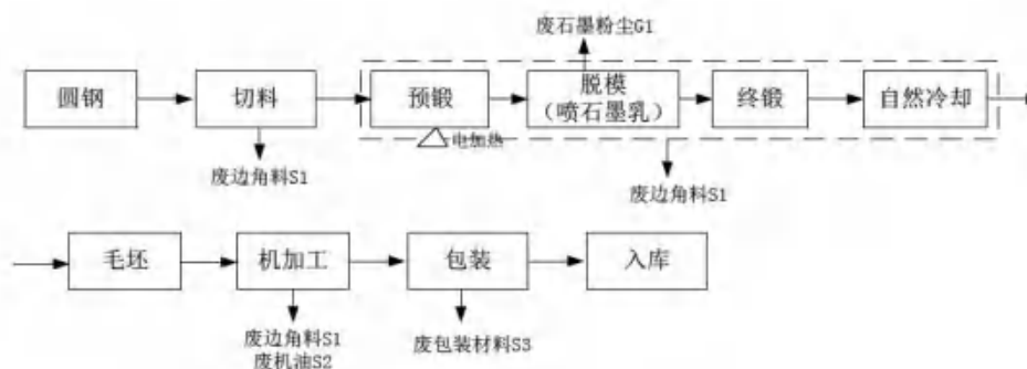
图 3-14 生产线工艺流程图
